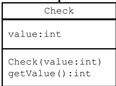
実装クラス Check
